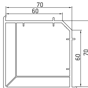
023 Уловый соединитель 90°
