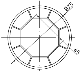
035 Соединитель-усилитель
