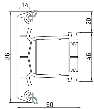
003 Импост 4-камерный
