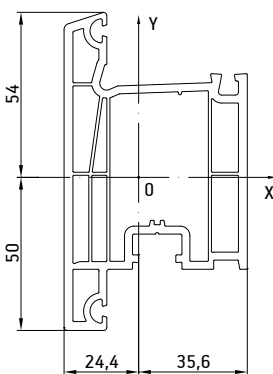
007 Дверная створка
