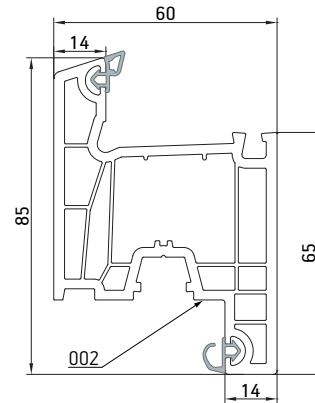
Створка 4-камерная 002
