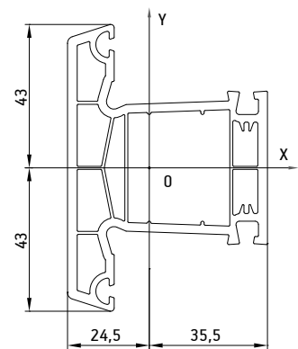
003 Импост
