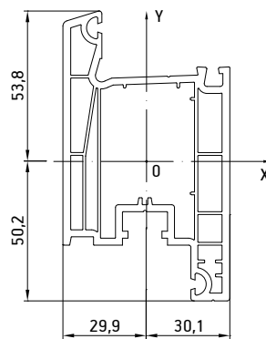
008 Дверная створка
