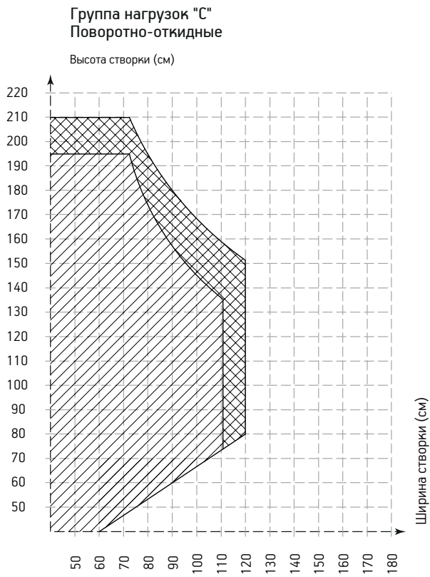
Створка 4-камерная
