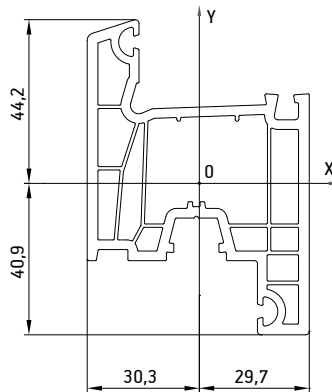
002 Створка
