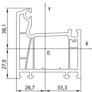
001 Рама
