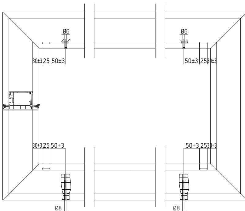
Ширина створки до 600мм
