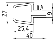
012 Штульп 60 мм
