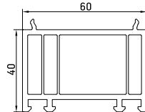
Н-соединитель рамы 024
