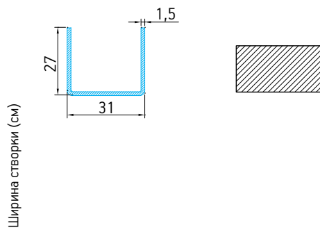
Створка 4-камерная с металлом U31/27/1,5
