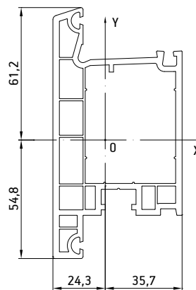
036 Дверная створка
