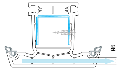
вертикальный импост
