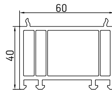
013 Расширитель рамы 40/60
