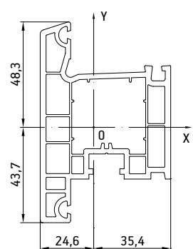
056 Дверная створка
