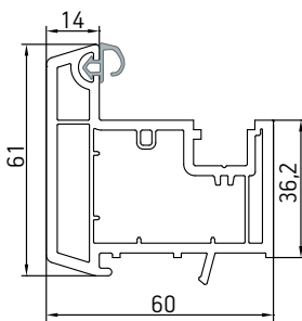
012 Штульп 60 мм
