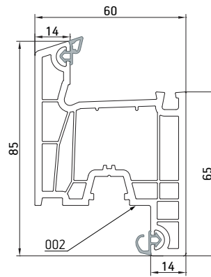
Створка 4-камерная
