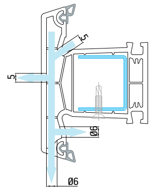
горизонтальный импост
